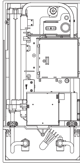
рис. 3 Установка прибора
