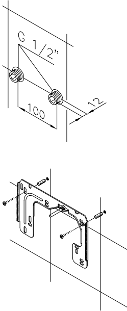
рис. 3 Установка прибора
